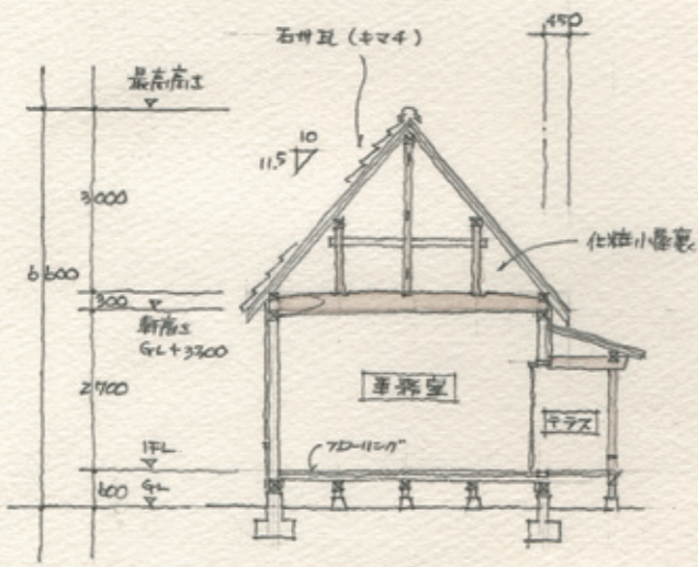
断面図 1/100
