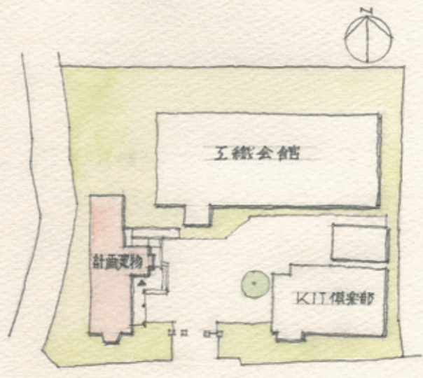
配置図 1/400
