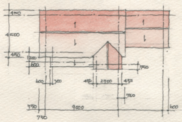
屋根伏図 1/200
