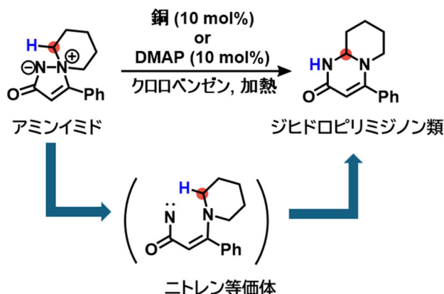
図4 予想された中間体を用いた実験
