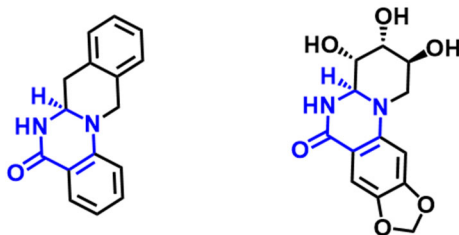
図1 抗がん活性を示すジヒドロピリミジノン類
