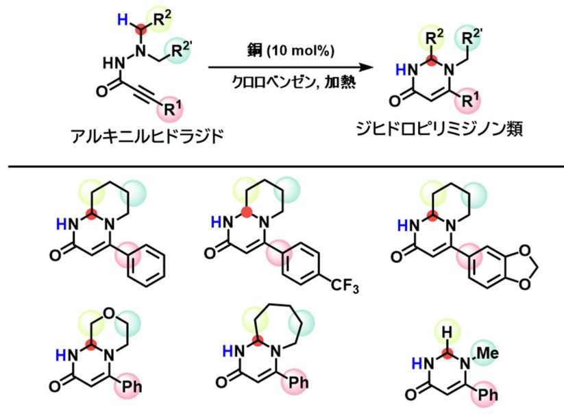
図3 反応式および合成した化合物の代表例
